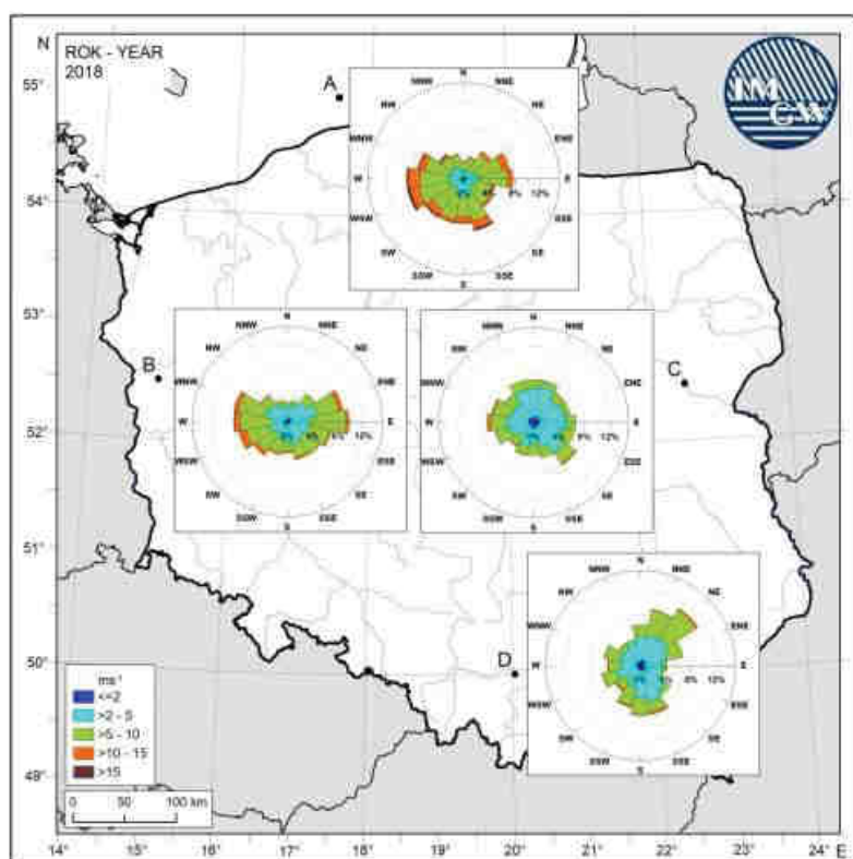
Rysunek 5. Kierunek oraz prędkość wiatru w punktach: A ( 55,0^{\circ}\text{N} , 17,5^{\circ}\text{E} ), B ( 52,5^{\circ}\text{N} , 15,0^{\circ}\text{E} ), C ( 52,5^{\circ}\text{N} , 22,5^{\circ}\text{E} ), D ( 50,0^{\circ}\text{N} , 20,0^{\circ}\text{E} ) 41
