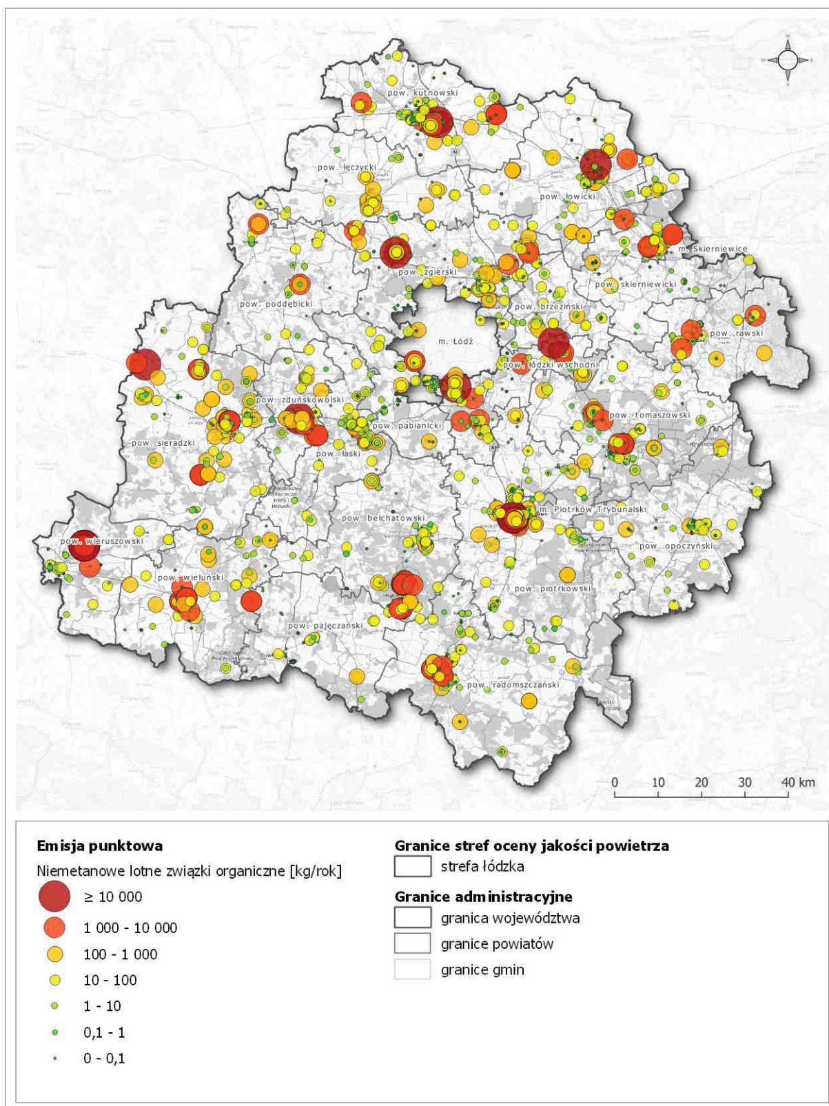
Rysunek 56. Rozmieszczenie emisji prekursorów ozonu (niemetaanowe lotne związki organiczne) z sektora przemysłu i energetyki na terenie strefy łódzkiej w 2018 roku 160
