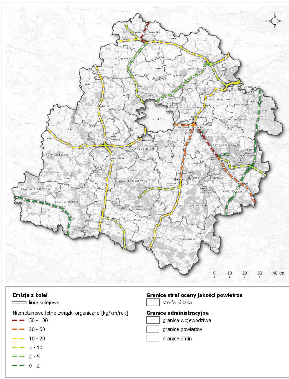
Rysunek 63. Rozmieszczenie emisji prekursorów ozonu (niemetanowe lotne związki organiczne) z kolei na terenie strefy łódzkiej w 2018 roku 167
