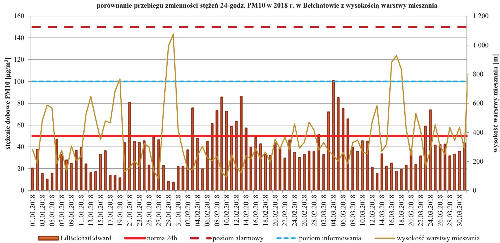
Rysunek 31. Porównanie przebiegu zmienności stężeń 24-godz. PM10 w I kwartale 2018 r. notowanych na stacjach pomiarowych w strefie łódzkiej z wysokością warstwy mieszanania 120
