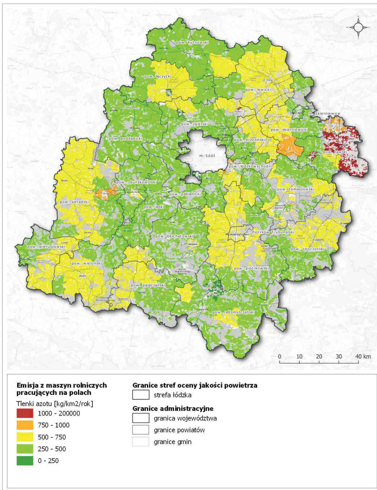
Rysunek 64. Rozmieszczenie emisji prekursorów ozonu (tlenki azotu NO x ) z maszyn rolniczych na terenie strefy łódzkiej w 2018 roku 168
