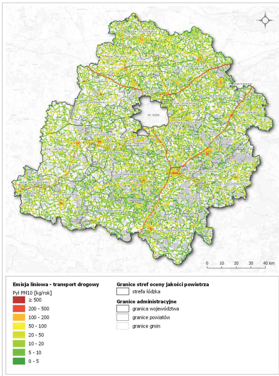
Rysunek 38. Rozmieszczenie emisji pyłu PM10 z sektora transportu drogowego na terenie strefy łódzkiej w 2018 roku 142
