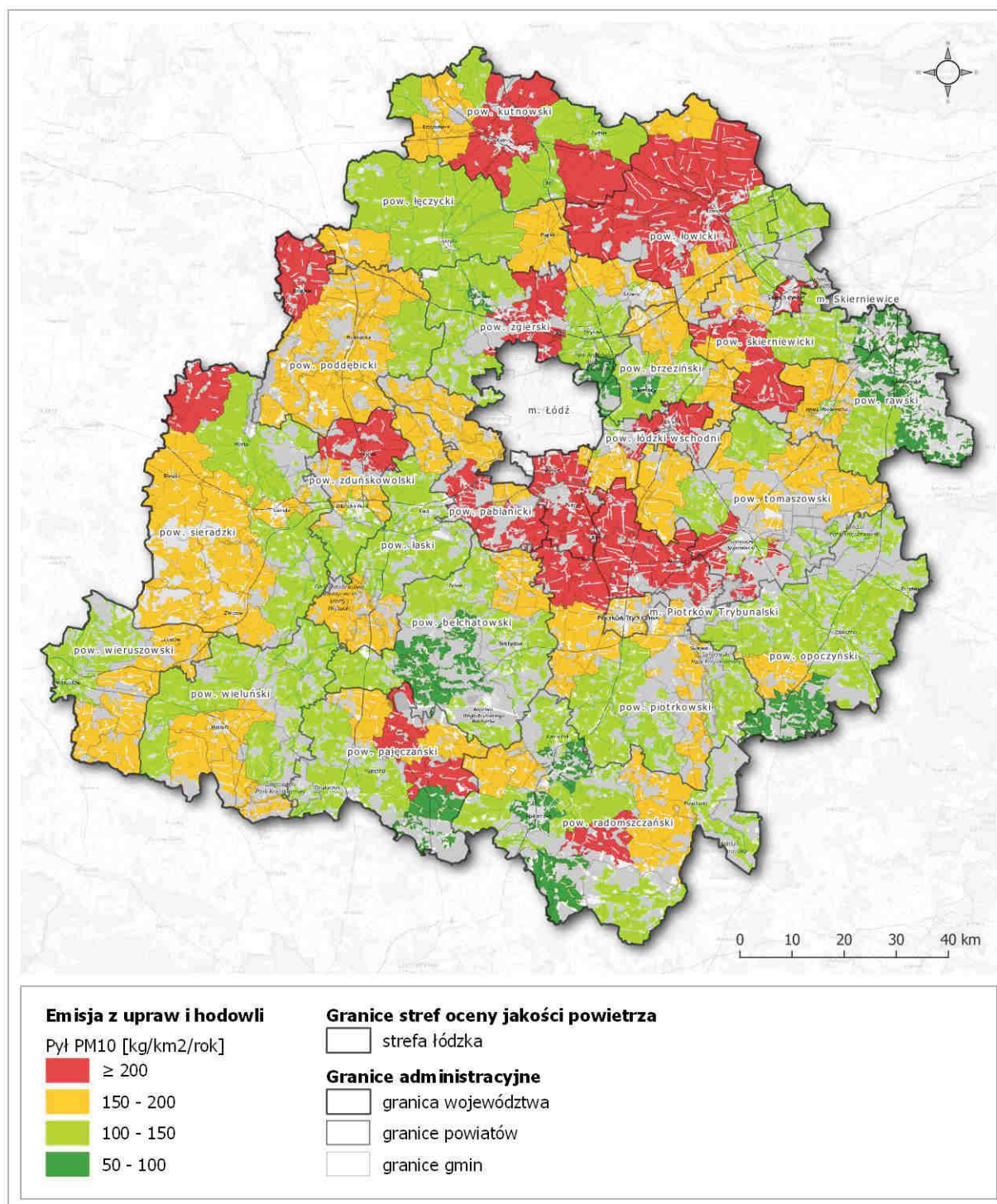
Rysunek 50. Rozmieszczenie emisji pyłu PM10 pochodzącej z sektora rolnictwa (uprawy i hodowla) na terenie strefy łódzkiej w 2018 roku 154
