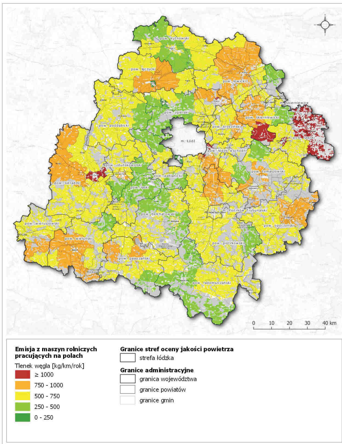
Rysunek 65. Rozmieszczenie emisji prekursorów ozonu (tlenek węgla CO) z maszyn rolniczych na terenie strefy łódzkiej w 2018 roku 169
