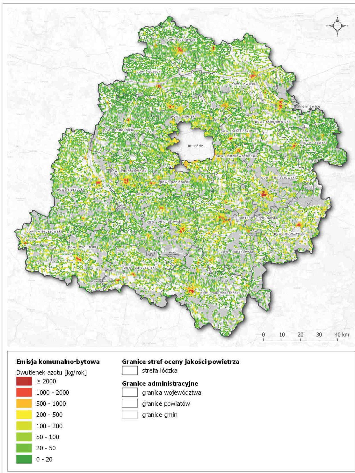
Rysunek 57. Rozmieszczenie emisji prekursorów ozonu (tlenki azotu NO x ) z sektora komunalno-bytowego na terenie strefy łódzkiej w 2018 roku 161
