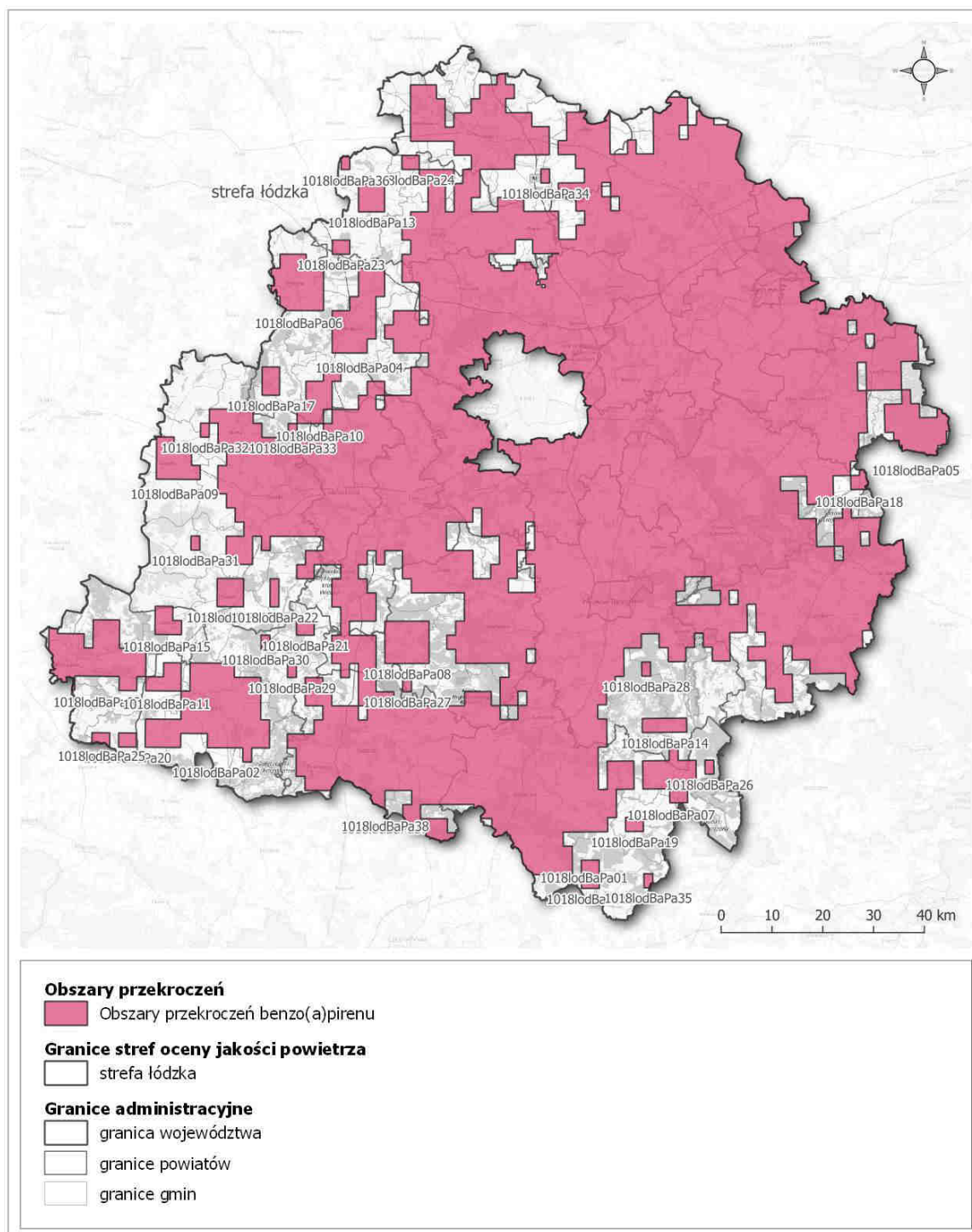
Rysunek 20. Obszary przekroczeń poziomu docelowego benzo(a)pirenu na terenie strefy łódzkiej w 2018 roku 73
