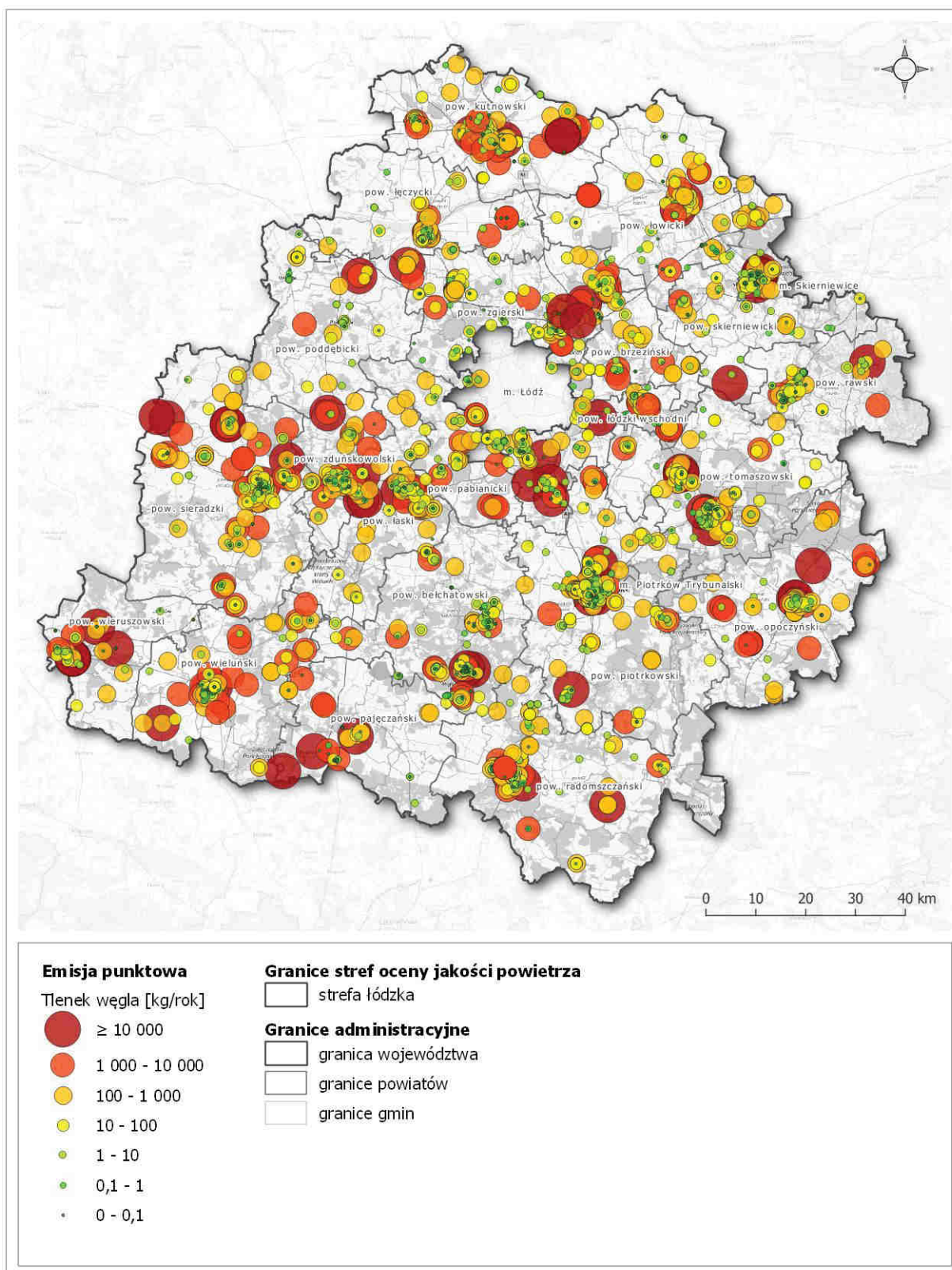
Rysunek 55. Rozmieszczenie emisji prekursorów ozonu (tlenek węgla CO) z sektora przemysłu i energetyki na terenie strefy łódzkiej w 2018 roku 159
