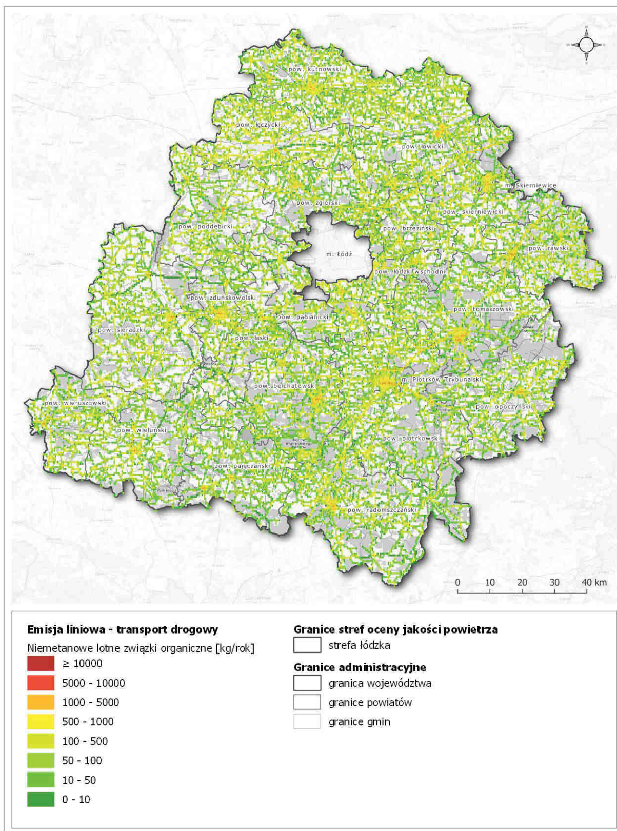
Rysunek 60. Rozmieszczenie emisji prekursorów ozonu (niemietanowe lotne związki organiczne) z sektora transportu drogowego na terenie strefy łódzkiej w 2018 roku 164
