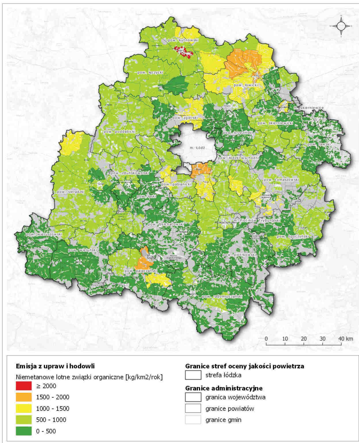
Rysunek 68. Rozmieszczenie emisji prekursorów ozonu (niemietanowe lotne związki organiczne) z rolnictwa (hodowla i uprawy) na terenie strefy łódzkiej w 2018 roku 172
