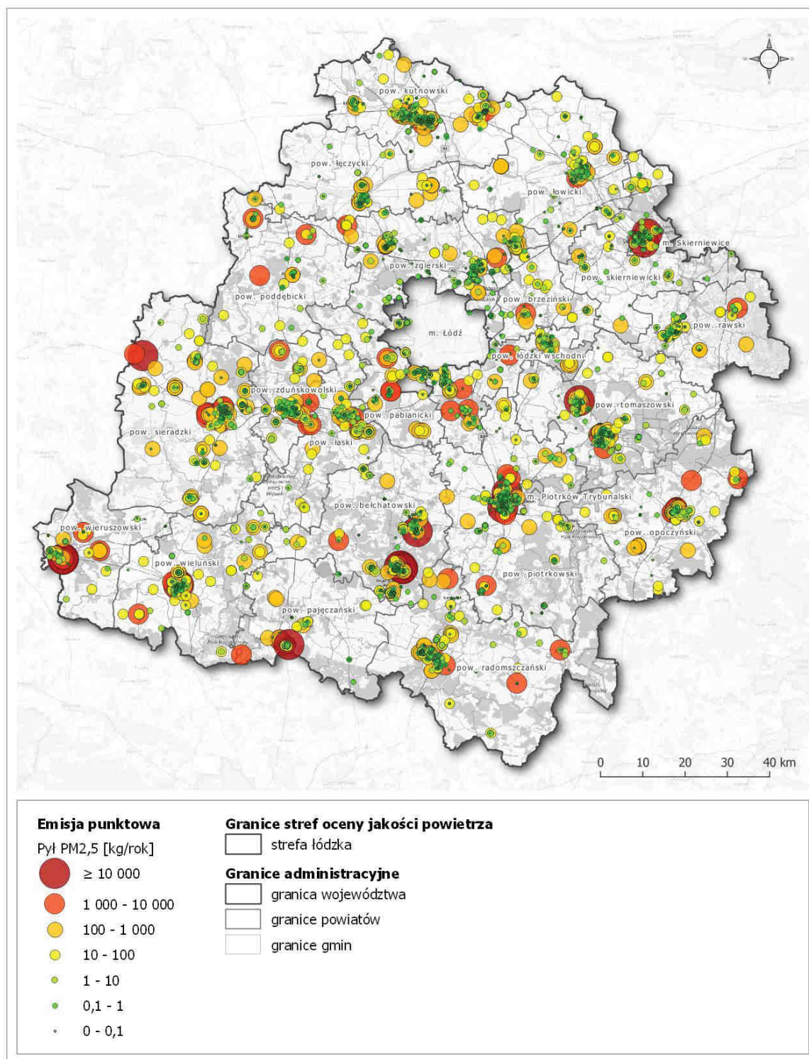
Rysunek 36. Rozmieszczenie emisji pyłu PM 2,5 z sektora przemysłu i energetyki na terenie strefy łódzkiej w 2018 roku 140
