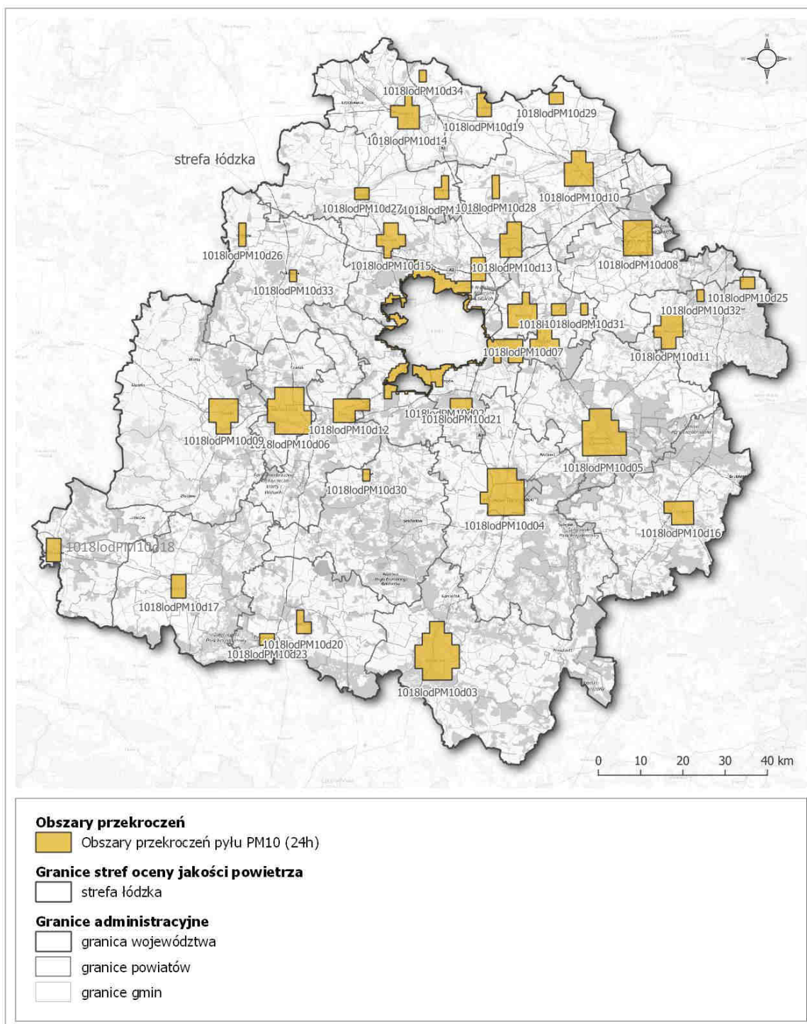
Rysunek 17. Obszary przekroczeń dopuszczanego poziomu dobowego pyłu zawieszony PM10 na terenie strefy łódzkiej w 2018 roku 70
