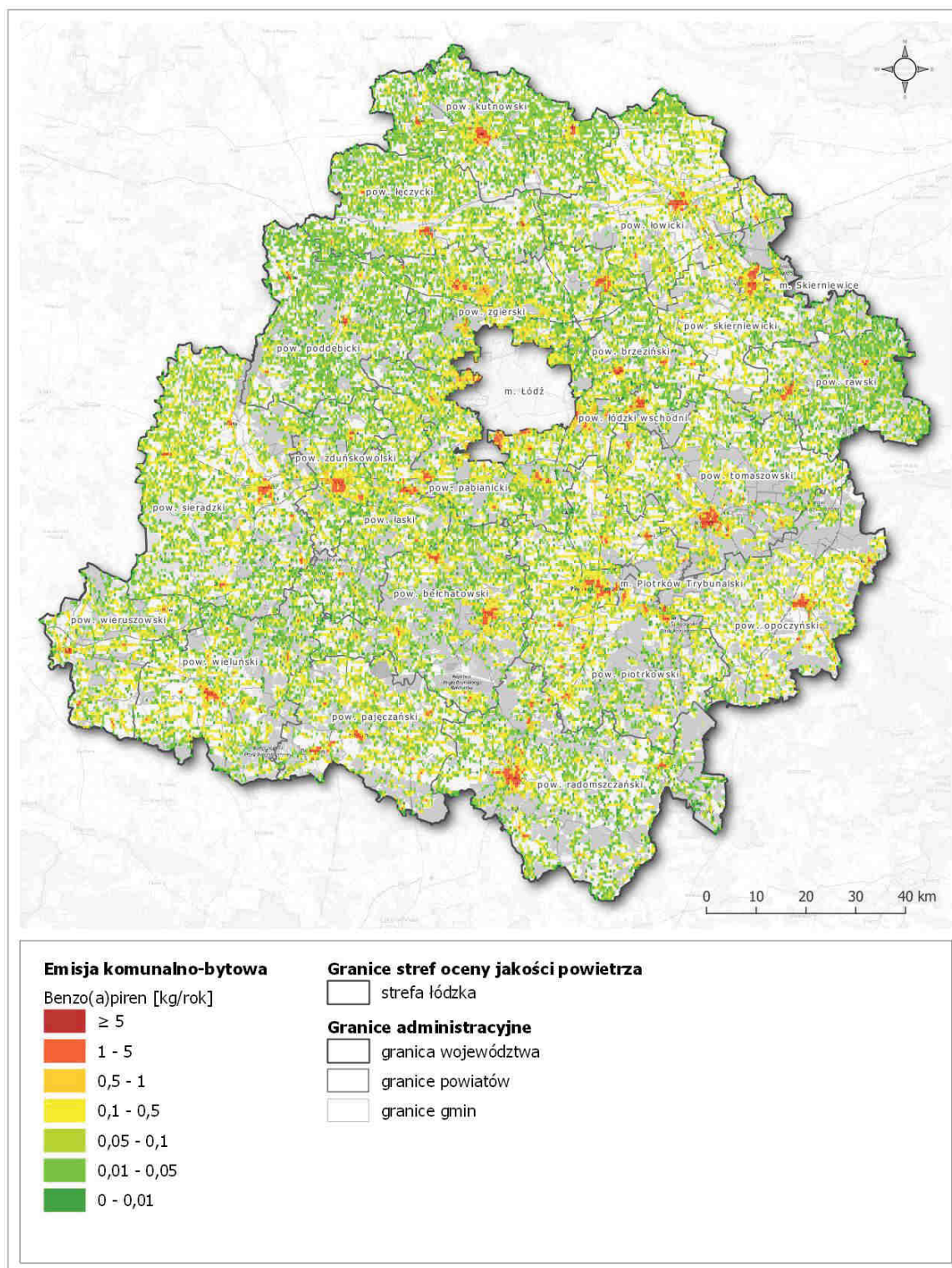
Rysunek 71. Rozmieszczenie emisji benzo(a)pirenu z sektora komunalno-bytowego na terenie strefy łódzkiej w 2018 roku 175
