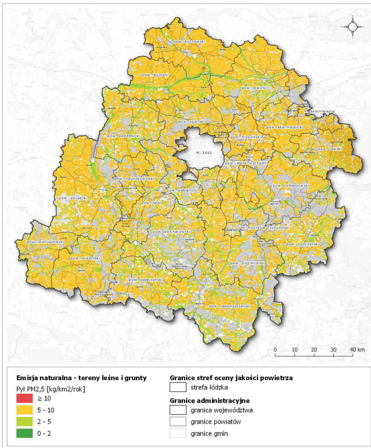
Rysunek 53. Rozmieszczenie emisji pyłu PM 2,5 pochodzącej z lasów i gruntów na terenie strefy łódzkiej w 2018 roku 157
