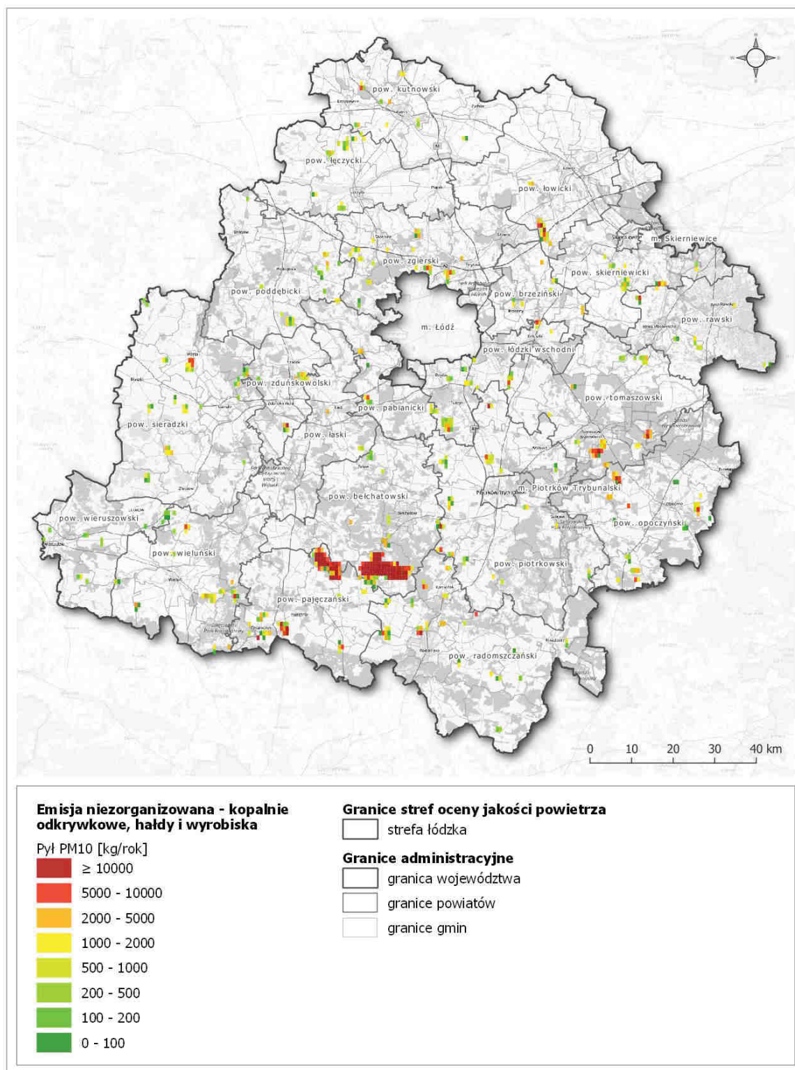
Rysunek 46. Rozmieszczenie emisji niezorganizowanej pyłu PM10 (hałdy i wyrobiska) na terenie strefy łódzkiej w 2018 rok 150
