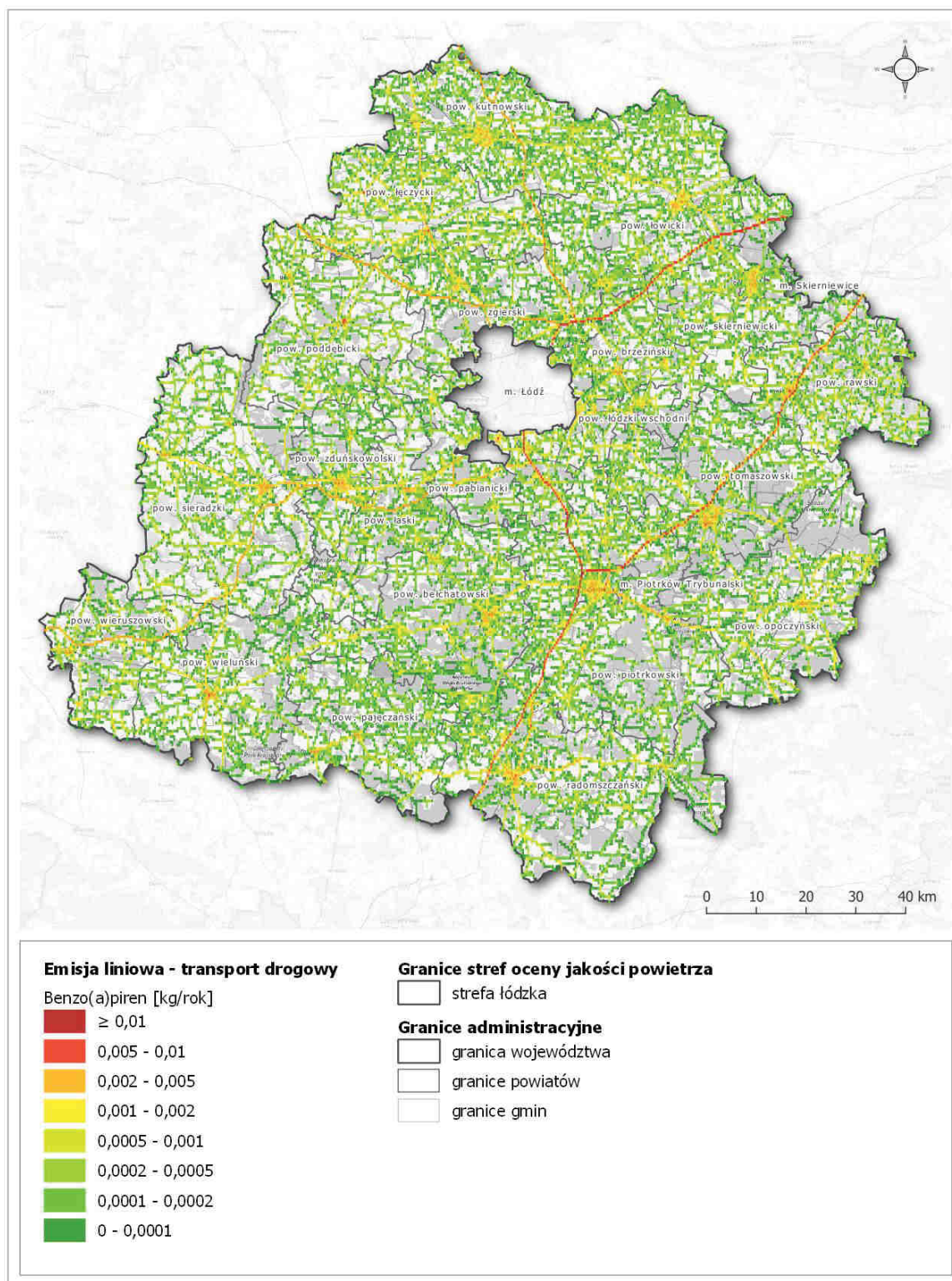
Rysunek 40. Rozmieszczenie emisji benzo(a)pirenu z sektora transportu drogowego na terenie strefy łódzkiej w 2018 roku 144
