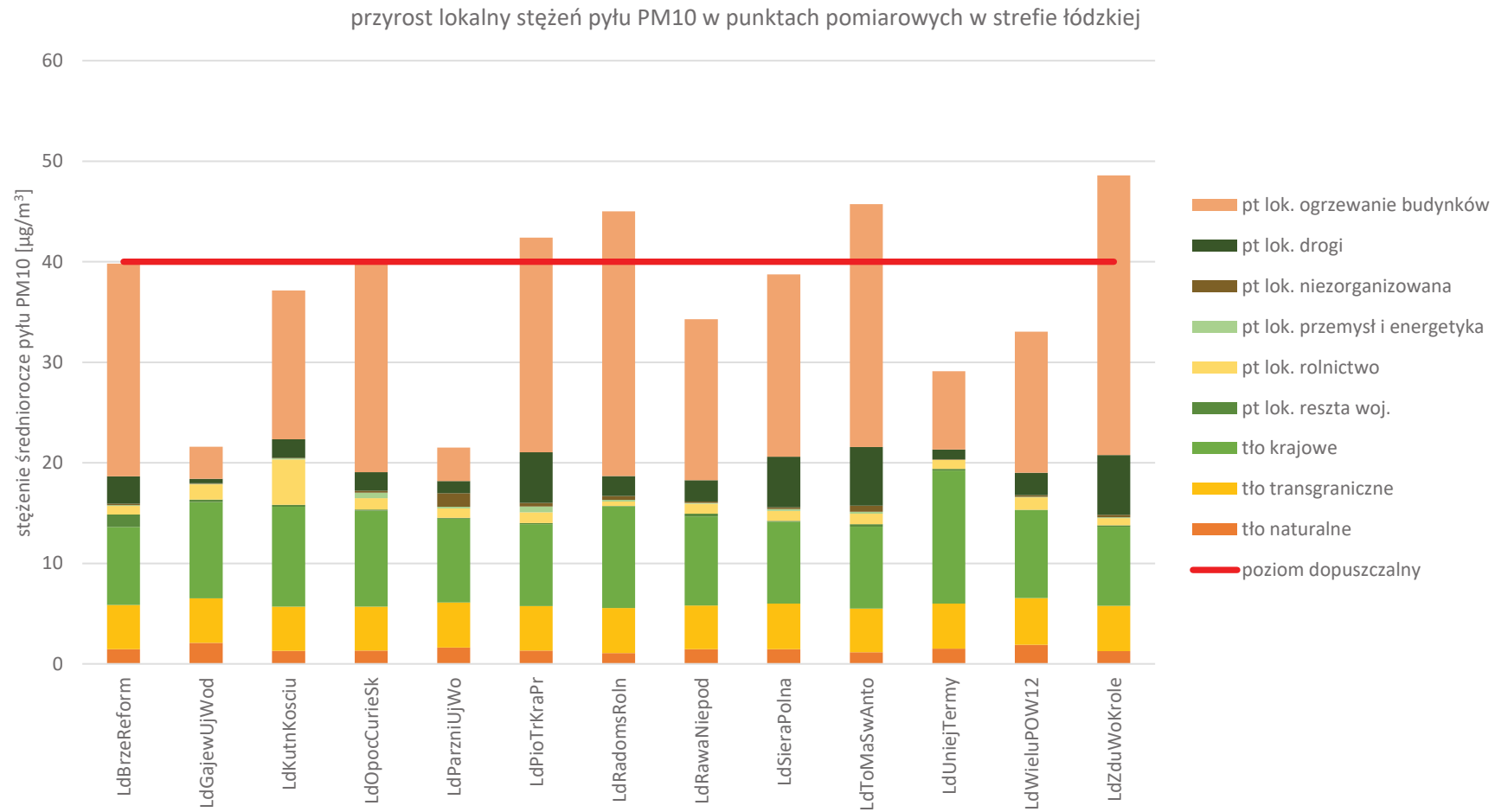
Rysunek 23. Prezentacja poziomów tła regionalnego oraz lokalnego przyrostu stężeń dla pyłu PM10 w punktach pomiarowych w strefie łódzkiej w 2018 roku 80
