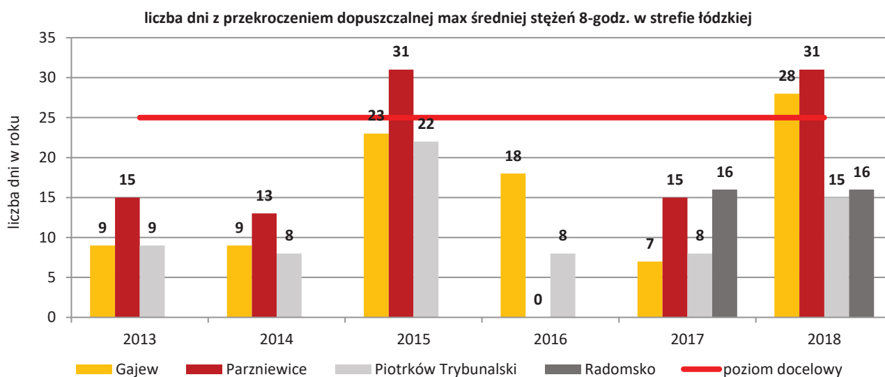
Rysunek 13. Liczba dni z przekroczeniem dopuszczalnej maksymalnej ośmiogodzinnej średnie kroczącej dla ozonu w punktach pomiarowych w strefie łódzkiej w latach 2013-2018
