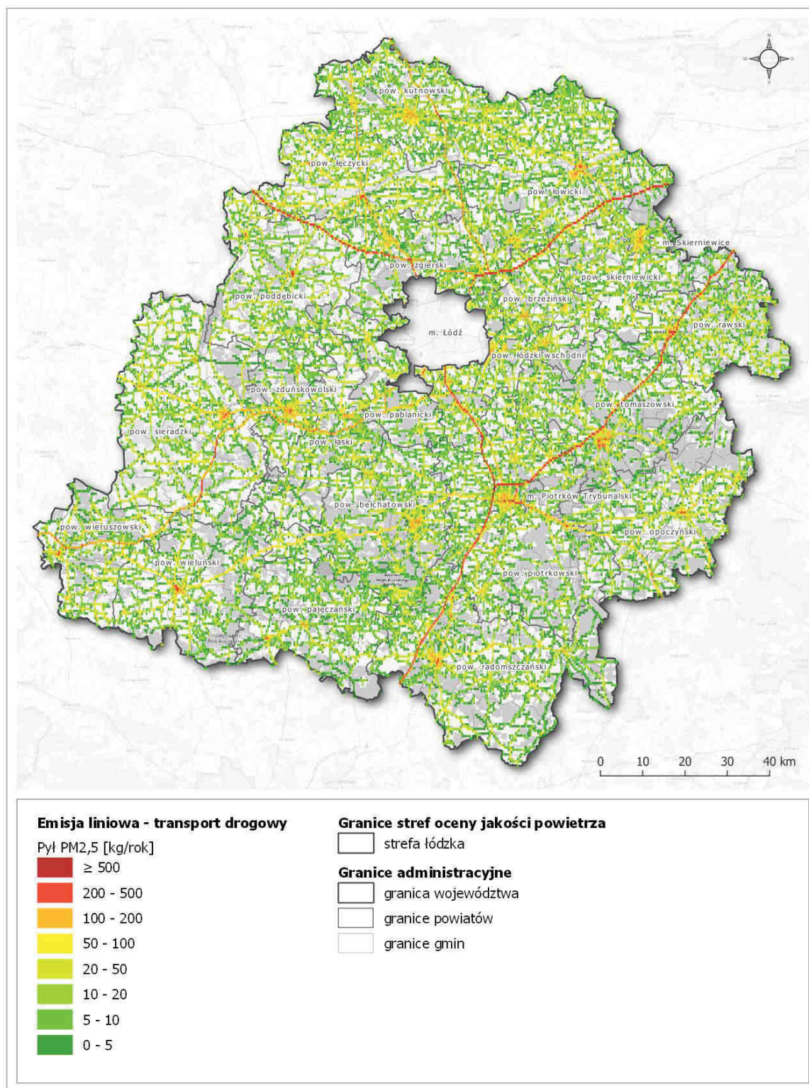
Rysunek 39. Rozmieszczenie emisji pyłu PM 2,5 z sektora transportu drogowego na terenie strefy łódzkiej w 2018 roku 143
