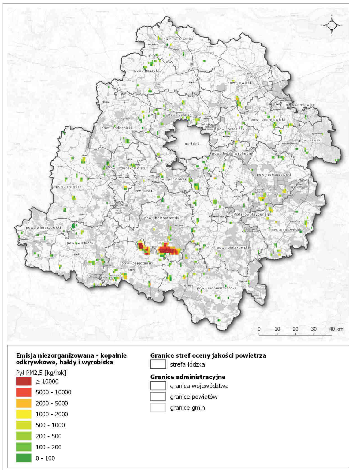
Rysunek 47. Rozmieszczenie emisji niezorganizowanej pyłu PM 2,5 (hałdy i wyrobiska) na terenie strefy łódzkiej w 2018 rok 151
