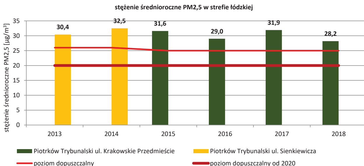
Rysunek 11. Wyniki pomiarów stężeń średniorocznych pyłu PM 2,5 w latach 2013-2018 w strefie łódzkiej 59
