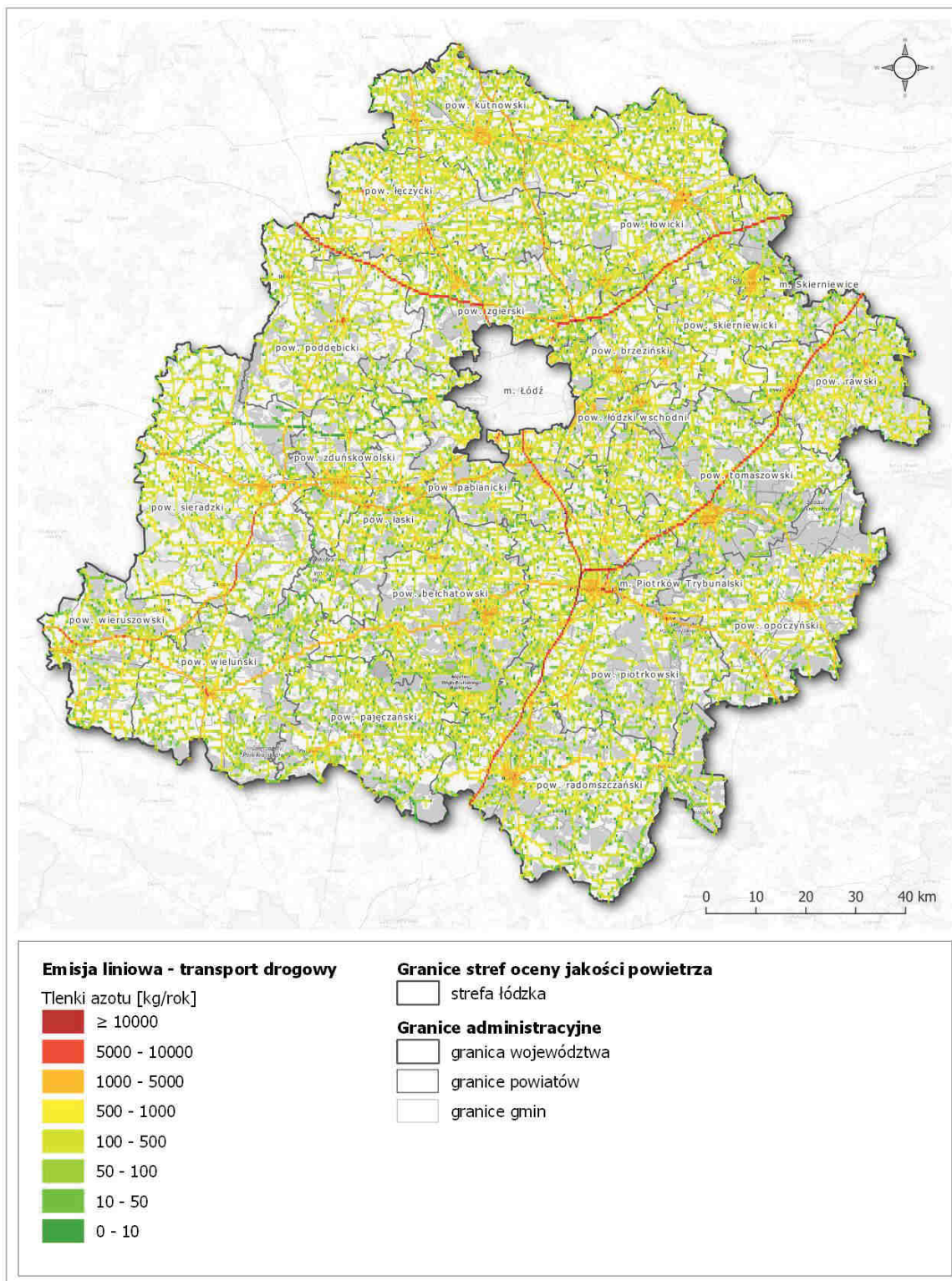
Rysunek 58. Rozmieszczenie emisji prekursorów ozonu (tlenki azotu NO_x ) z sektora transportu drogowego na terenie strefy łódzkiej w 2018 roku 162
