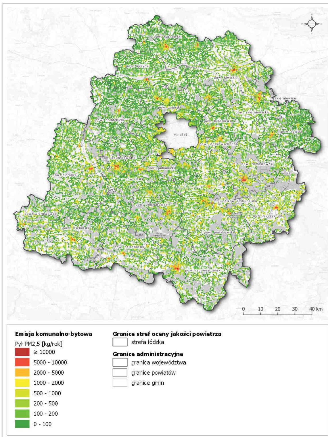
Rysunek 70. Rozmieszczenie emisji pyłu PM 2,5 z sektora komunalno-bytowego na terenie strefy łódzkiej w 2018 roku 174
