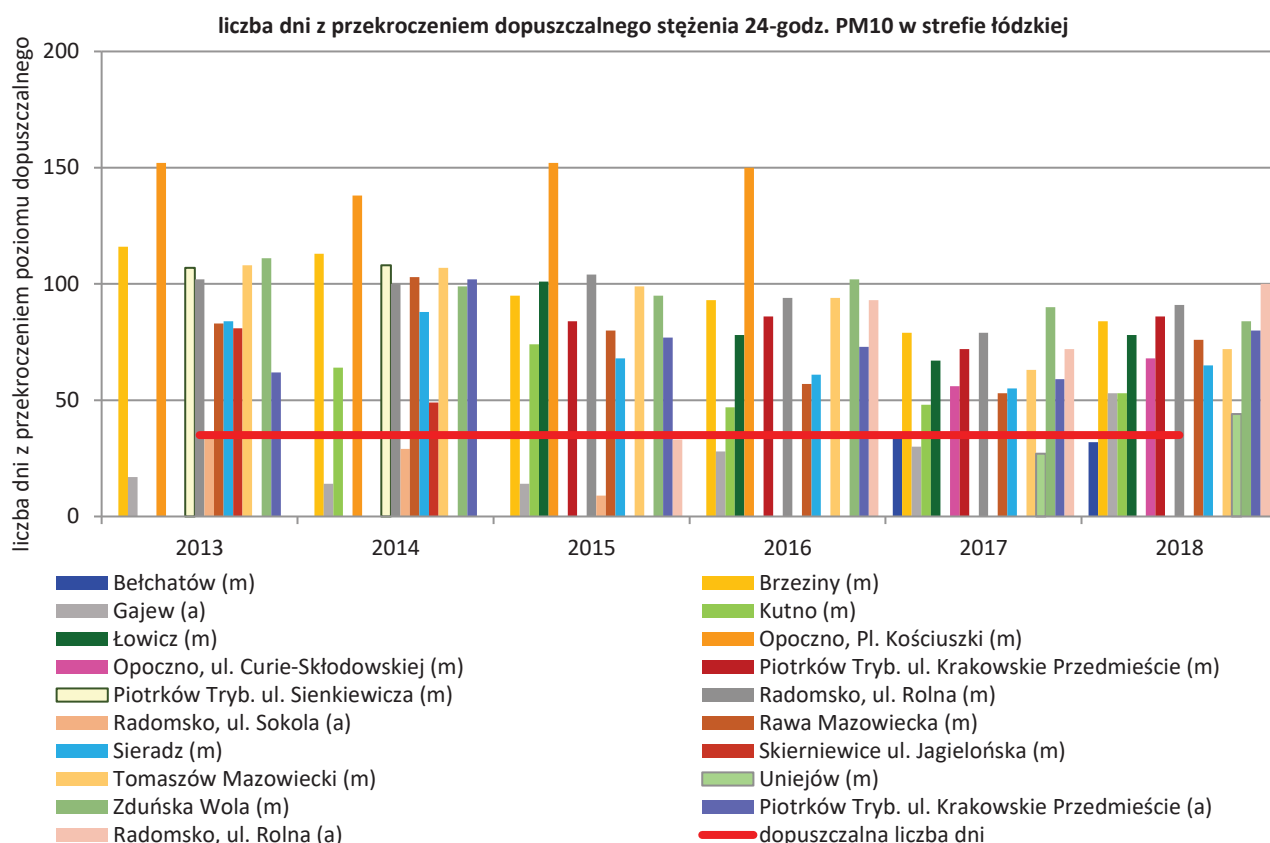
Rysunek 10. Liczba dni z przekroczeniem poziomu dopuszczalnego 24-godzinny pyłu PM10 w latach 2013-2018 w punktach pomiarowych w strefie łódzkiej 55
