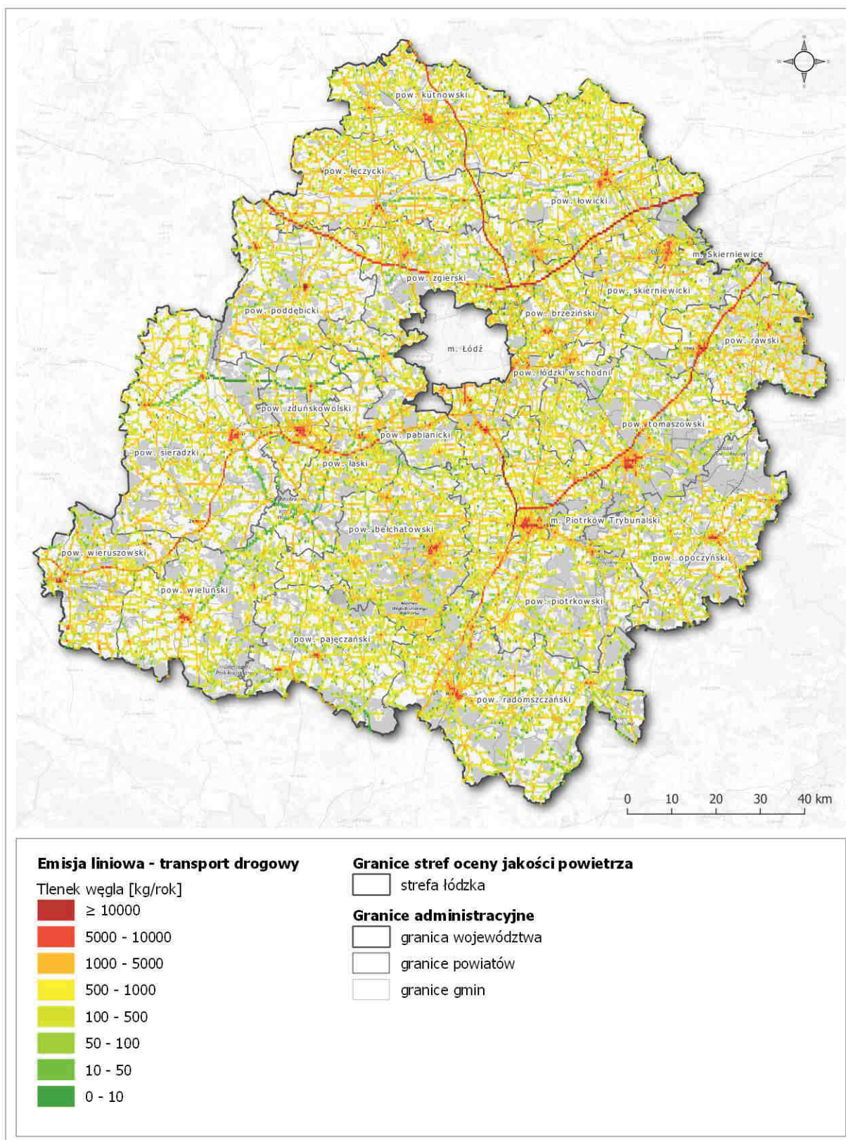
Rysunek 59. Rozmieszczenie emisji prekursorów ozonu (tlenek węgla CO) z sektora transportu drogowego na terenie strefy łódzkiej w 2018 roku 163
