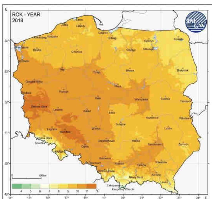
Rysunek 2. Średnia roczna temperatura powietrza w roku 2018 38
